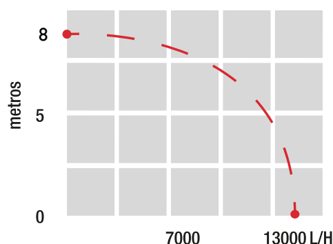
DIAGRAMA CAPACIDAD CAUDAL
